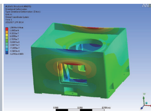
座位分析結果 (Z方向變形)
