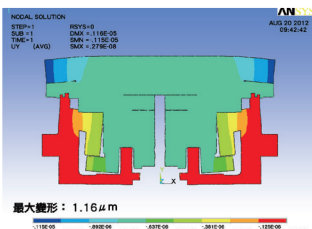
旋轉盤分析結果 (轉盤Y方向變形)
