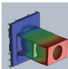
主軸座位移分析
