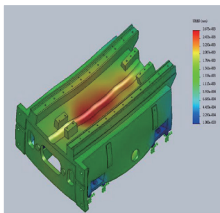
底座位移分析
