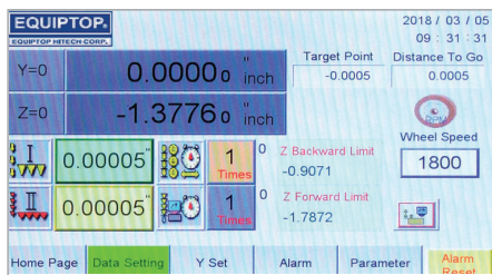
工件研磨條件尺寸設定
