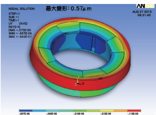
方向變形Y圓盤導軌 (旋轉盤分析結果)
