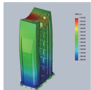
動柱位移分析
